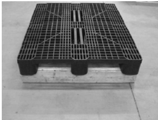
Configuration du test : Vue de devant
