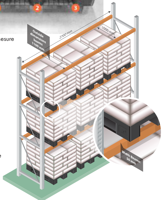
Crémaillère palette
